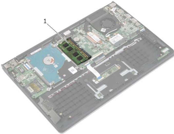
1 메모리 모듈
